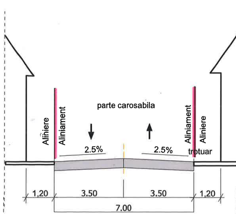
PROFIL DRUM EXISTENT
